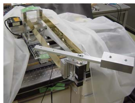
柔軟リンクに搭載されたロボットアーム
